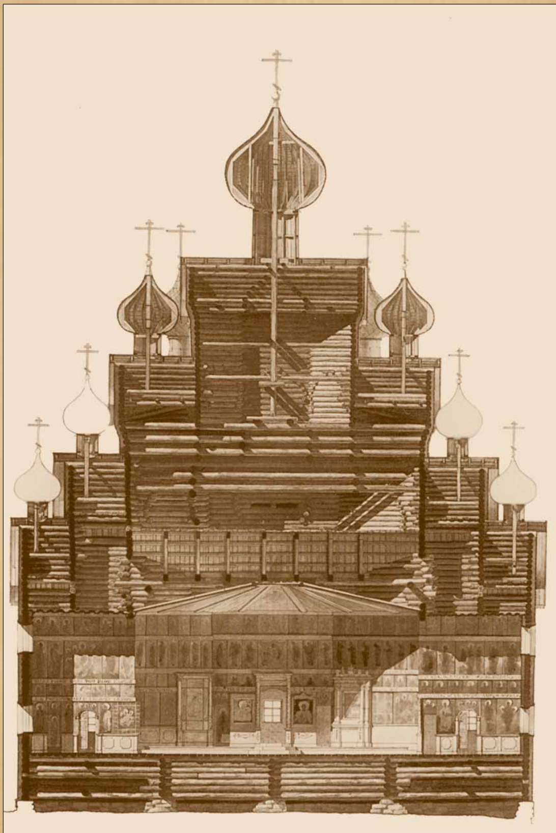
Покровская церковь близ Вытегры. Реконструкция. Разрез
